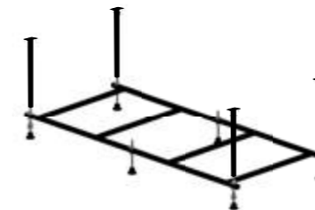
Каркас для ванны Calipso CAL1775i92
